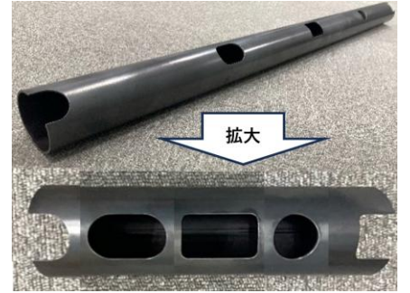
各種穴明け・切欠き加工(エンドミル)
