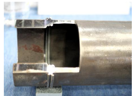
摩擦圧接
