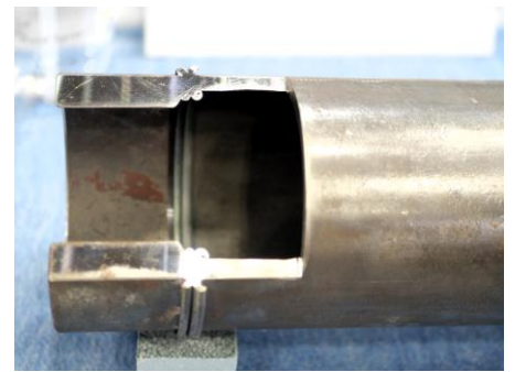
摩擦圧接
