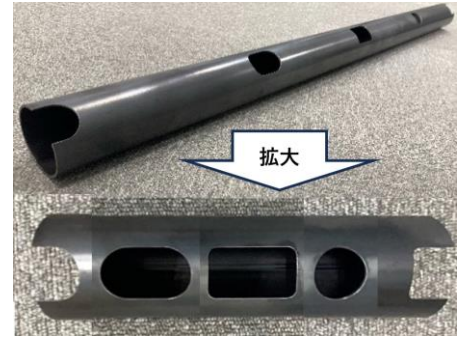
各種穴明け・切欠き加工(エンドミル)
